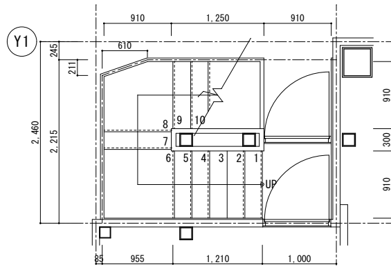
1階階段平面図 1/50
