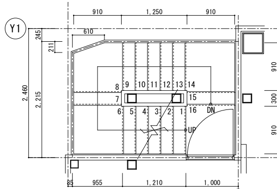
2～4階階段平面図 1/50
