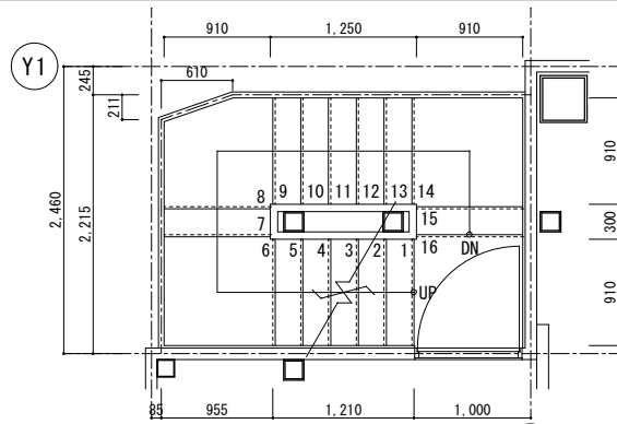
5階階段平面図 1/50
