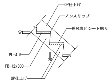
A部分詳細図 1/30
