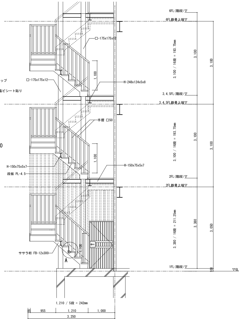
階段断面詳細図 1/50
